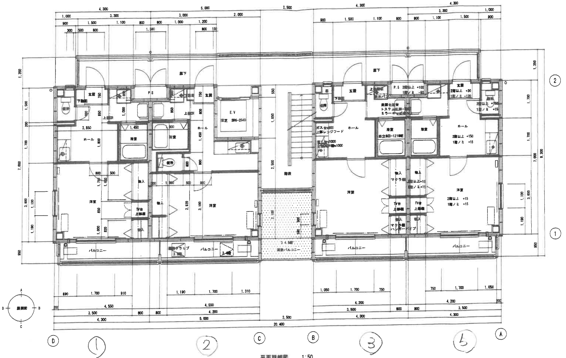
平面詳細図 1:50
