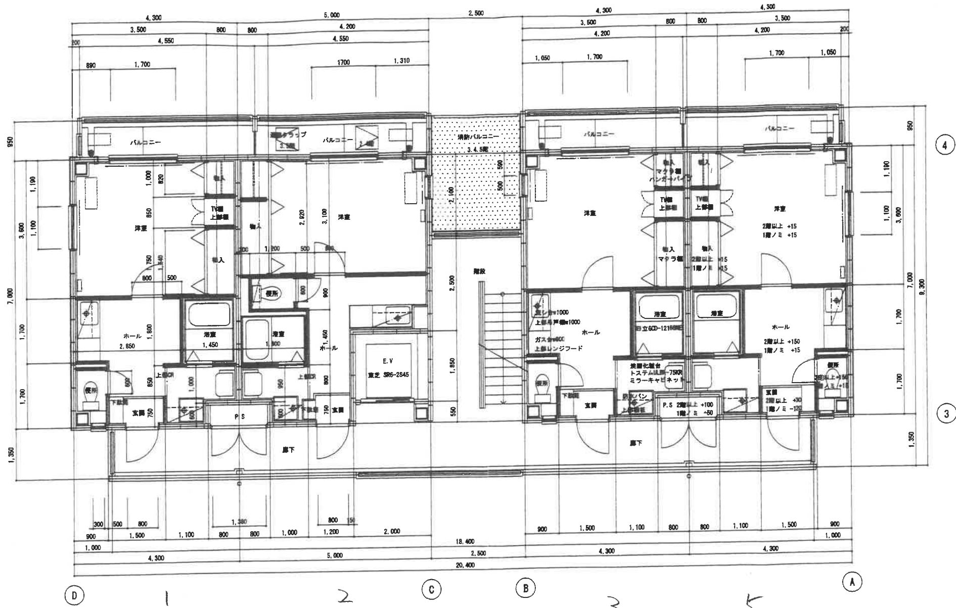
平面詳細図 1:50
