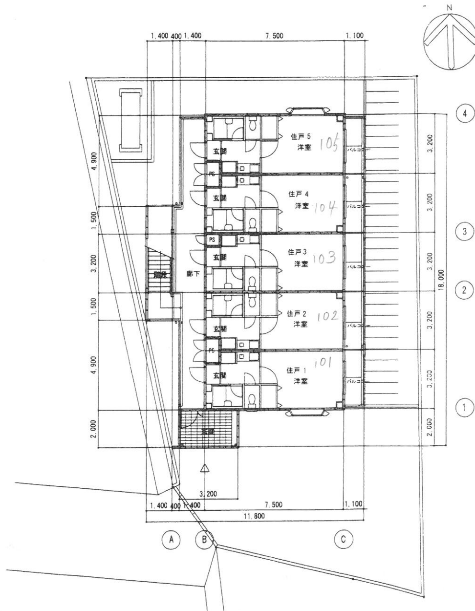
1階平面図 1:100
