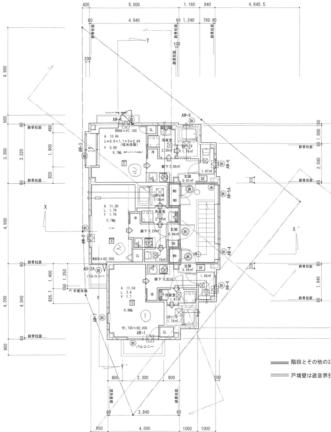
[ 4階平面図 1/100 ]
