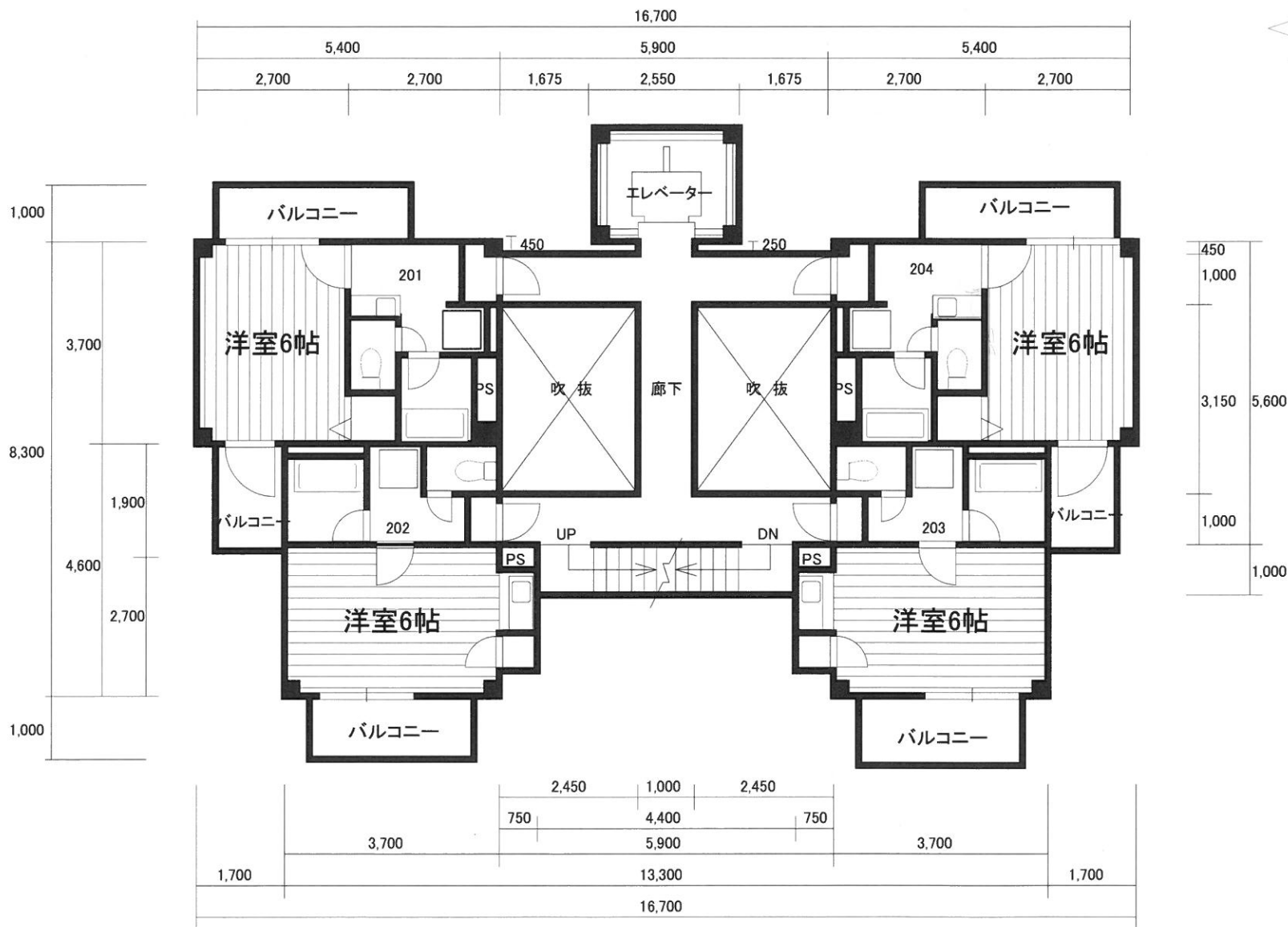
2階～6階平面図
